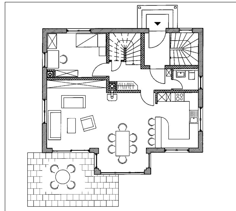
Das in Markelfingen erstellte Energie-Einspar-Haus verfügt über eine nutzbare Fläche von 214 Quadratmetern.
