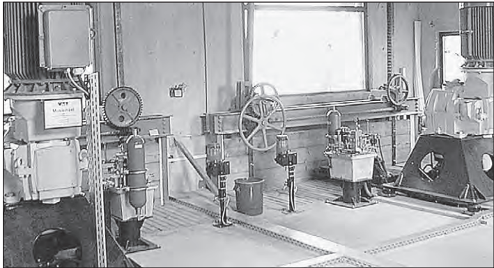
Hier kommt der Strom her: Ein Blick in den Turninenraum des neuen Wasserkraftwerks auf der Singener Musikinsel.
