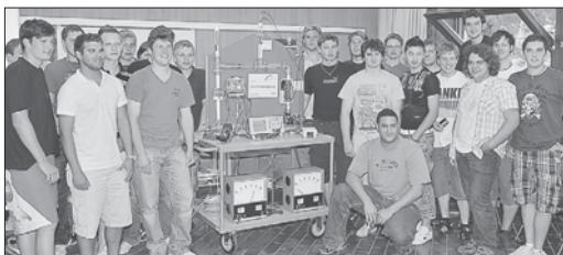
Ein Gerät zur Durchflussmessung und Durchflussregelung haben die Mechatroniker im dritten Lehrjahr an der Hohentwiel-Gewerbeschule konstruiert und gebaut. Letzte Woche konnte es präsentiert werden. swb-Bild: of
