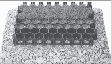
Die Rasenschutzwaben lassen Wasser in den Boden versickern und entsiegeln damit die Oberfläche. swb-Bild: epr/Ritter
