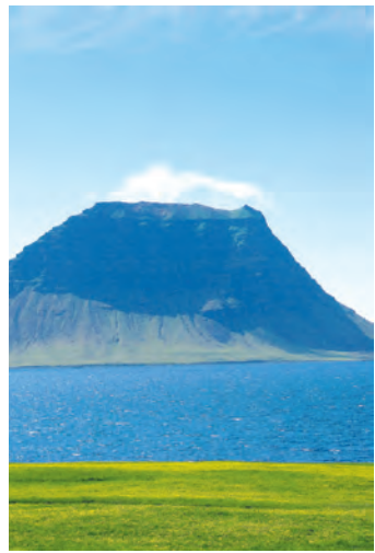
Eines hat Island mit dem Hegau gemein: seine Vulkane. swb-Bild: Museumsverein
