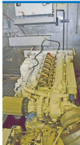
Motor: Der 500-PS-Motor der MS Seestern. Normale Fahrtgeschwindigkeit ist 14 km/h, Höchstgeschwindigkeit 28 km/h.
