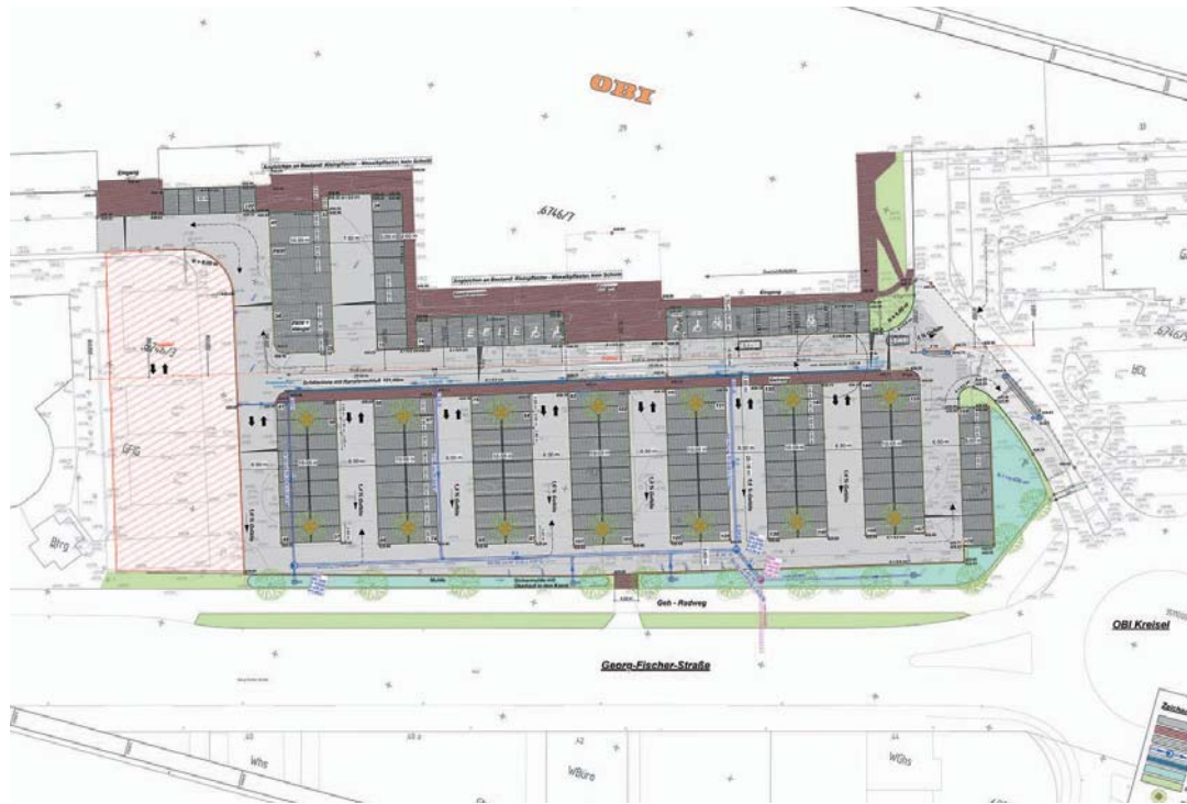
So wird der OBI-Parkplatz nach den Umbauarbeiten im kommenden Frühjahr angeordnet sein. Dann können die Kunden und Besucher direkt von der Erschließungsstraße in die dann neu angelegten Parkreihen einfahren. sub-Graphik: Ingenieurbüro Baur
