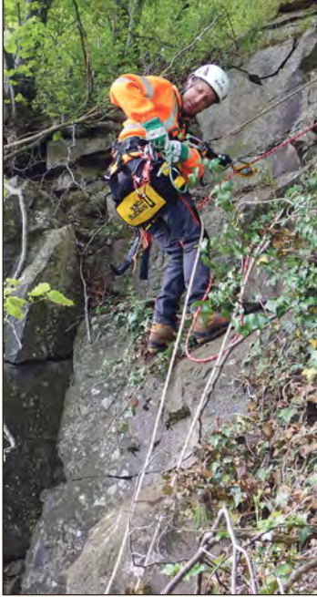
Ein Mitarbeiter des Landesamts für Geologie, Rohstoffe und Bergbau (LGRB) untersucht den betroffenen Fels am Hohentwiel (Foto: LGRB).
