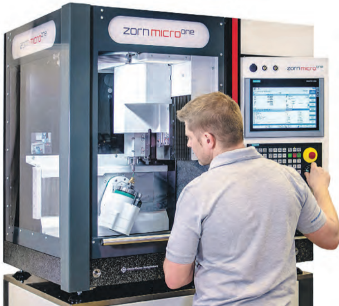
ZORN microone-5-Achs-Bearbeitungszentrum
