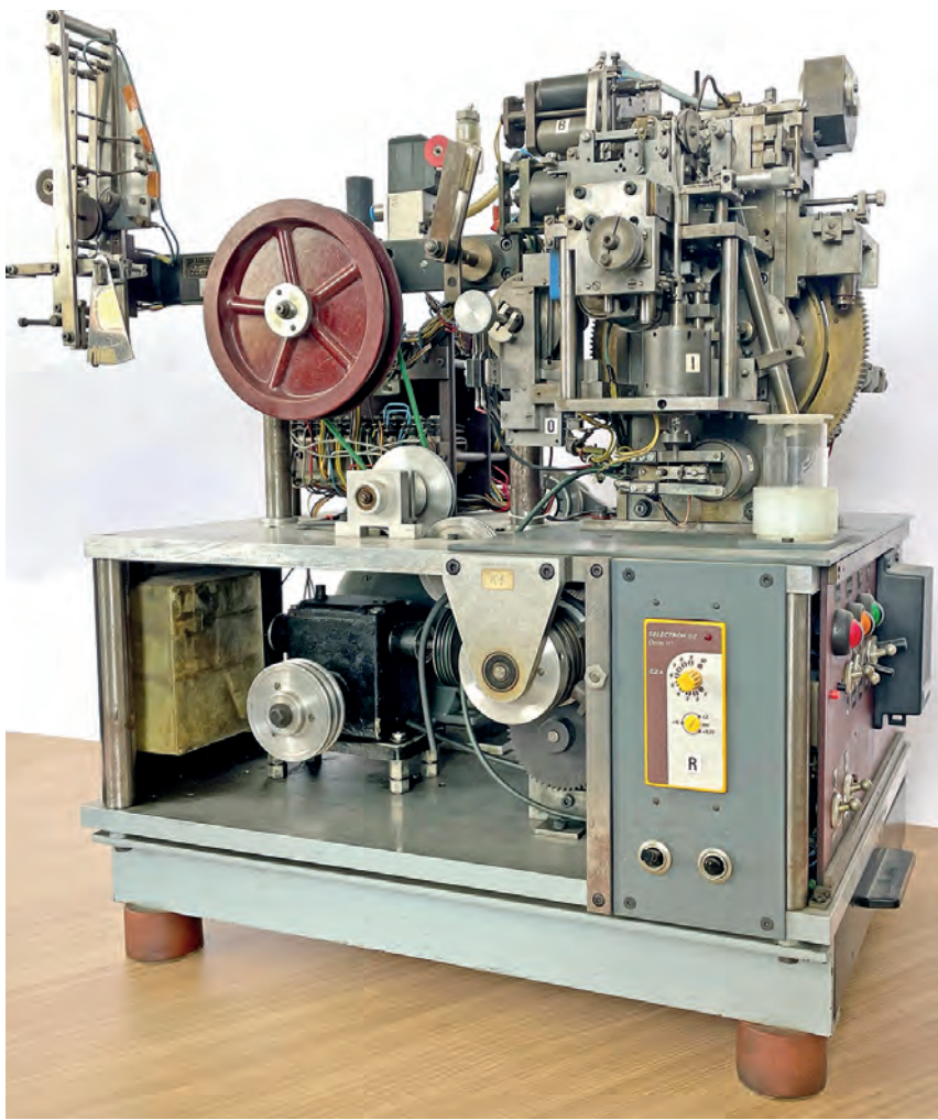
Wendelmaschine zum Wickeln von Glühwendeln aus den 1960er Jahren; in Betrieb bis 2005.
