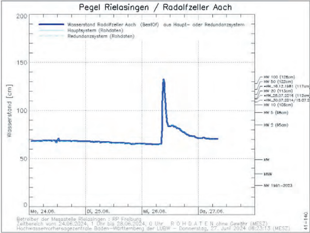
Die Pegelkurve der Aach vom Mittwoch erinnert an ein Erdbeben. Innerhalb weniger Minuten wurde die Marke des „HQ100“ (hundertjähriges Hochwasser) erreicht. swb-Bild: RP Freiburg/HVZ/LUBW
