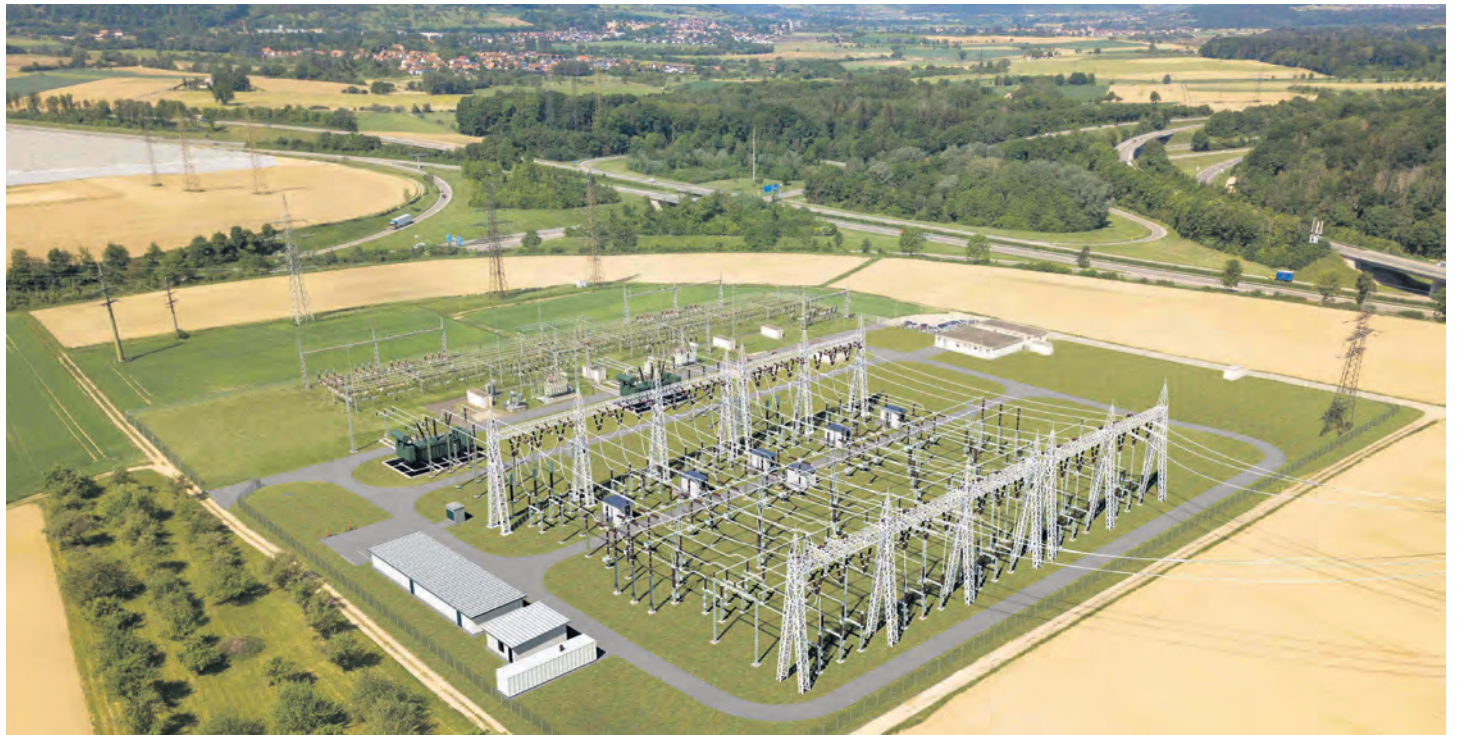
Von oben gesehen fast schon zierlich wird die Planung des neuen Umspannwerks bei Singen-Beuren der Transnet BW, das bis 2026 in Betrieb gehen soll. sub-Bild: Transnet BW
