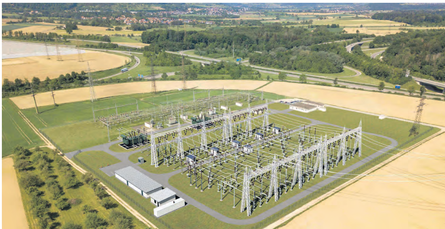
Von oben gesehen fast schon zierlich wird die Planung des neuen Umspannwerks bei Singen-Beuren der Transnet BW, das bis 2026 in Betrieb gehen soll.
