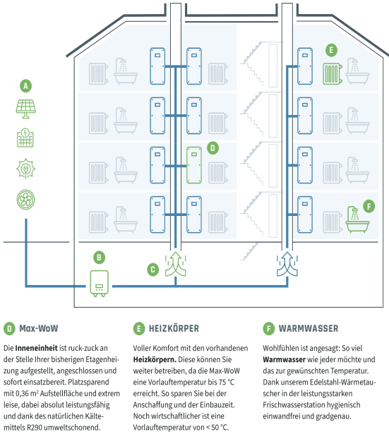
So funktioniert die neue Etagenwärmepumpe... swb-Bild: Becker Energie
